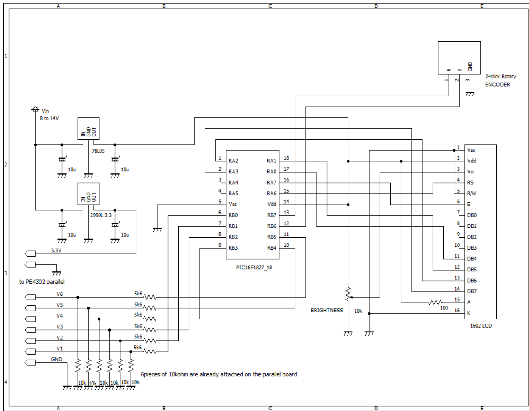
图1. Digital ATT Parallel回路图
